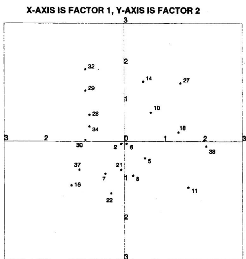
Figura 1. Representación bidimensional de los factores 1 y 2.
