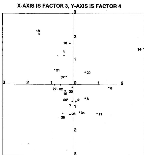
Figura 2. Representación bidimensional de los factores 3 y 4.
